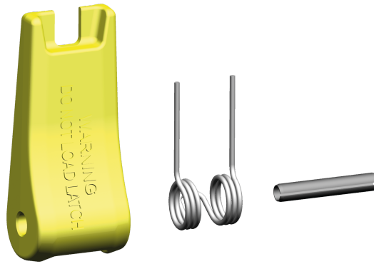
Oryginalne zdjęcie zestawu SFGW-B firmy pewag.
