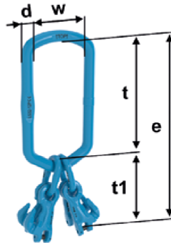
Rysunek VLSXK 4 G12 Plus z katalogu pewag, s. 25. Wymiary opisano w tabeli.
