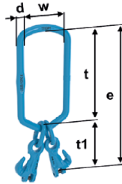
Rysunek VLSXK 2 G12 Plus z katalogu pewag, s. 24. Wymiary opisano w tabeli.
