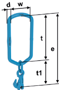
Rysunek VLSXK 1 G12 Plus z katalogu pewag, s. 23. Wymiary opisano w tabeli.
