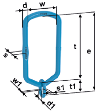
Rysunek VLS 1 G12 Plus z katalogu pewag, s. 18. Symbole odpowiadają wymiarom w tabeli.
