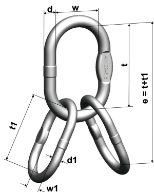
Rysunek VAWI: e = t + t1 . Wymiary d , t , w dotyczą ogniwa głównego, a d1 , t1 , w1 — ogniw przejściowych.
