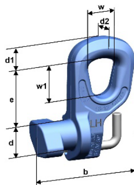
Schemat pewag CHWP. Oznaczenia odpowiadają tabeli wymiarów.
